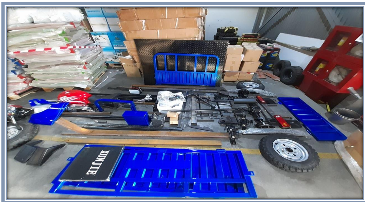
3-расм. Демонтаж қилинган уч ғилдиракли юк мотоцикли.
